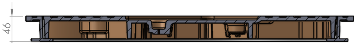
SECTION A-A SCALE 1 : 4
